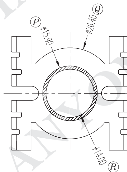
SEC. A-A
